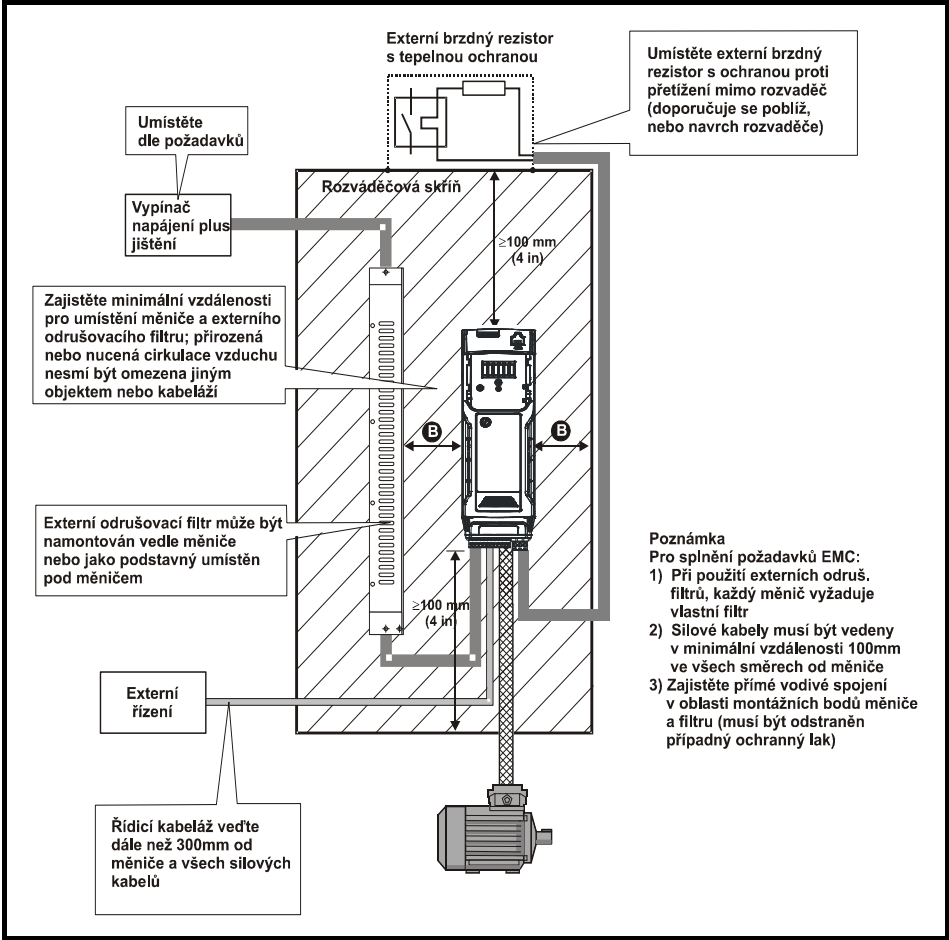
Obr. 3-14 Uspořádání rozváděče
