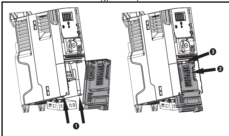
Obr. 3-6 Montáž volitelného SI modulu (typ. vel. 2 až 4)
