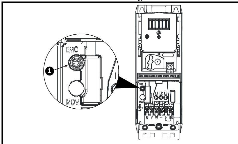
Obr. 3-16 Demontáž interního odrušovacího filtru u typ. vel. 2
