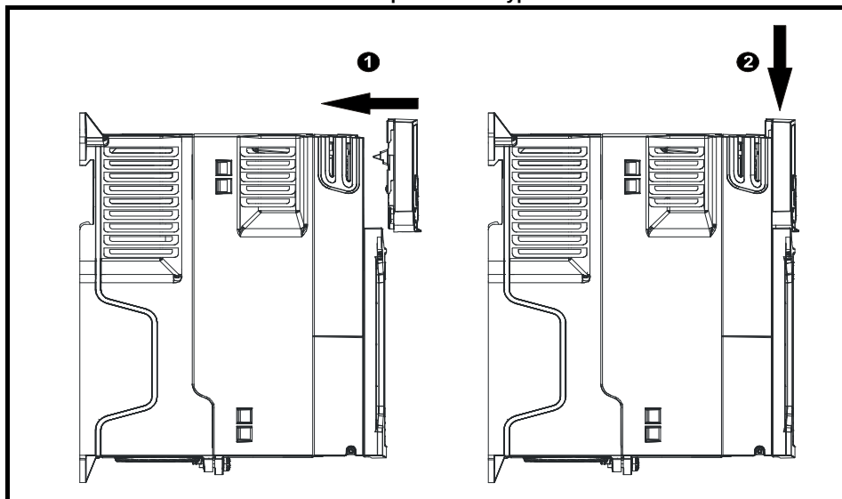
Obr. 3-12 Montáž a demontáž ovládacího panelu CI-Keypad
