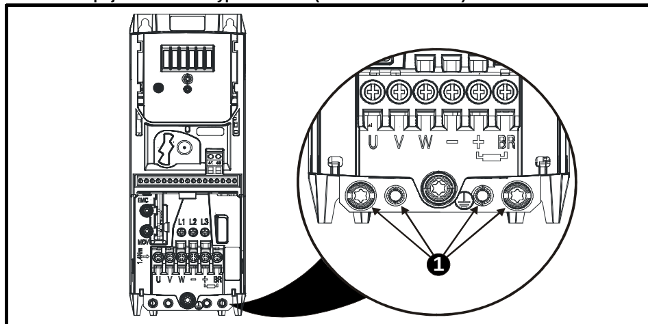
Obr. 4-5 Připojení zemnění - typ. vel. 1 až 4 (zobrazena velikost 2)
