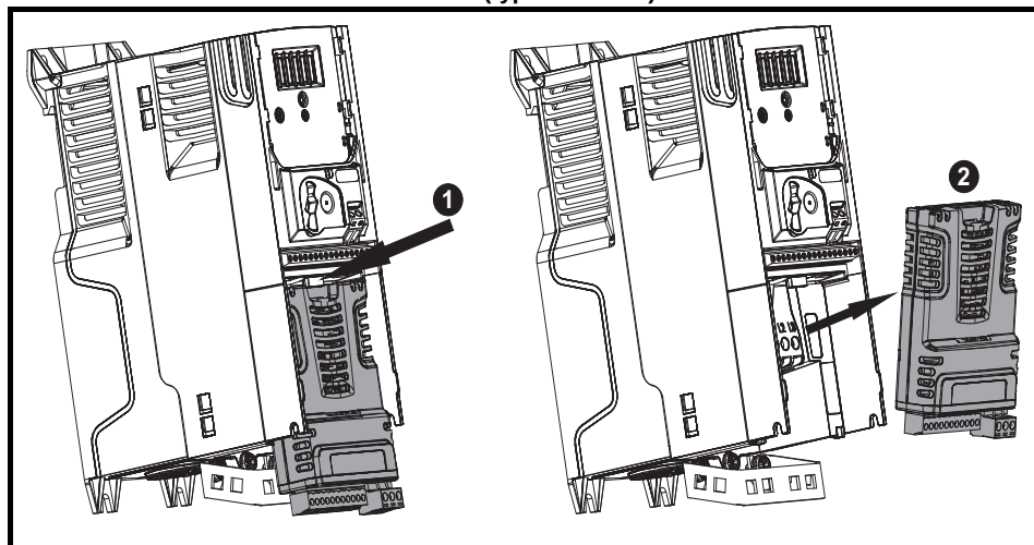
Obr. 3-7 Demontáž volitelného SI modulu (typ. vel. 2 až 4)
