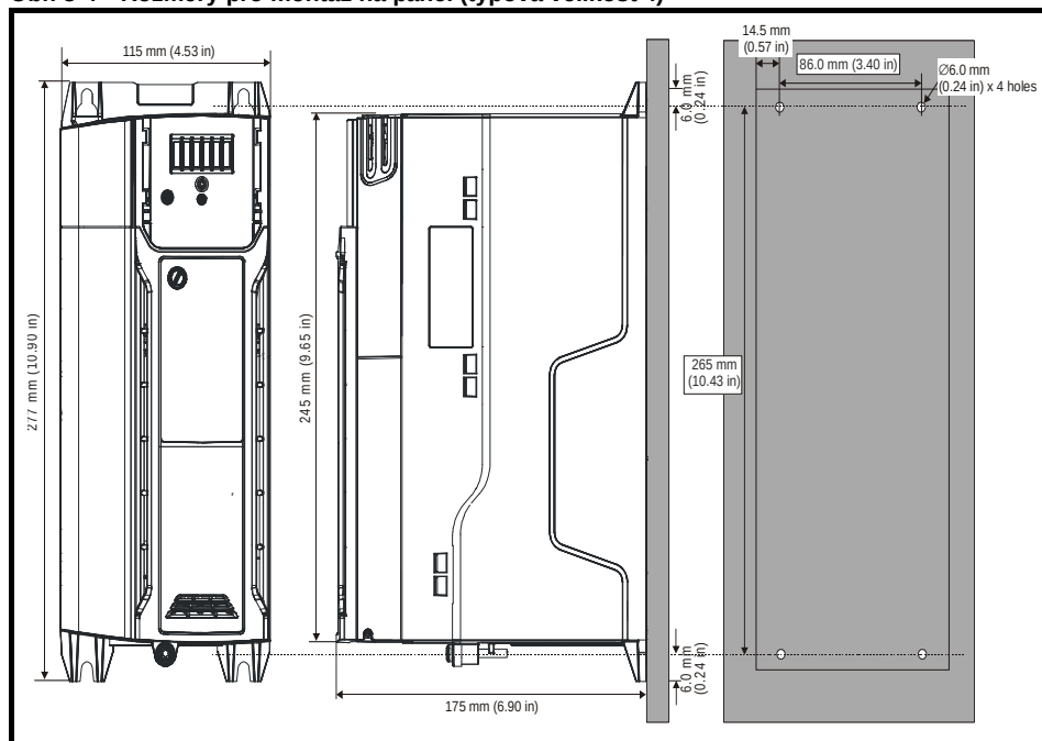
Obr. 3-4 Rozměry pro montáž na panel (typová velikost 4)
