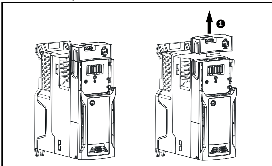
Obr. 3-9 Demontáž adaptéru AI-485
