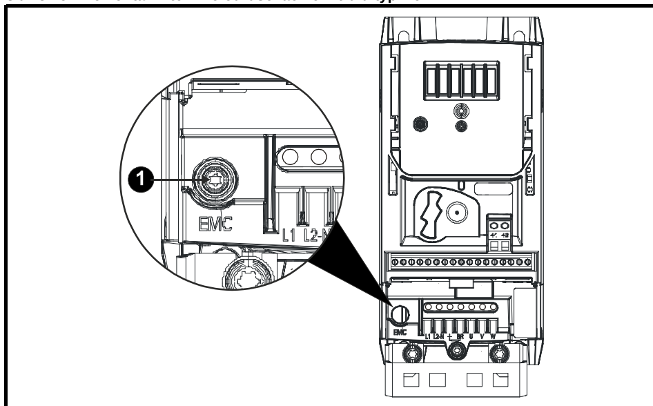
Obr. 3-15 Demontáž interního odrušovacího filtru u typ. vel. 1
