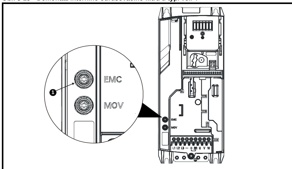
Obr. 3-18 Demontáž interního odrušovacího filtru u typ. vel. 4
