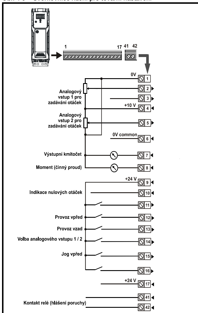
Obr. 4-6 Svorkovnice řízení pro tovární nastavení
