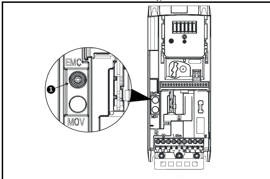
Obr. 3-17 Demontáž interního odrušovacího filtru u typ. vel. 3
