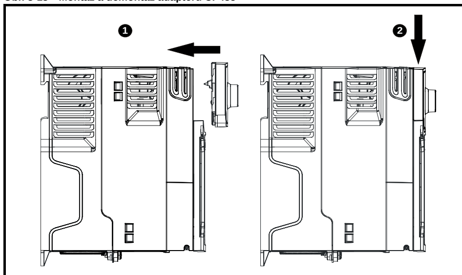
Obr. 3-13 Montáž a demontáž adaptéru CI-485
