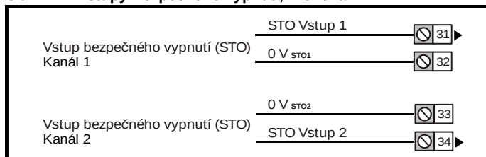
Obr. 4-7 Vstupy Bezpečného vypnutí, Blokování
