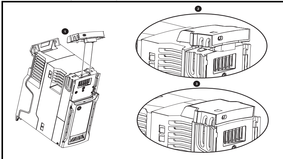
Obr. 3-10 Montáž adaptéru AI-Backup
